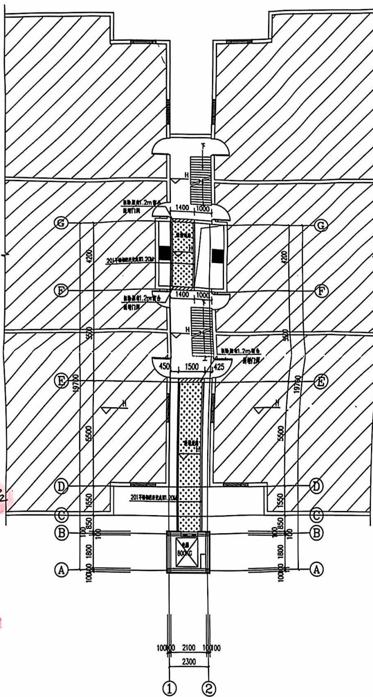
增设电梯三~八层平面示意图
