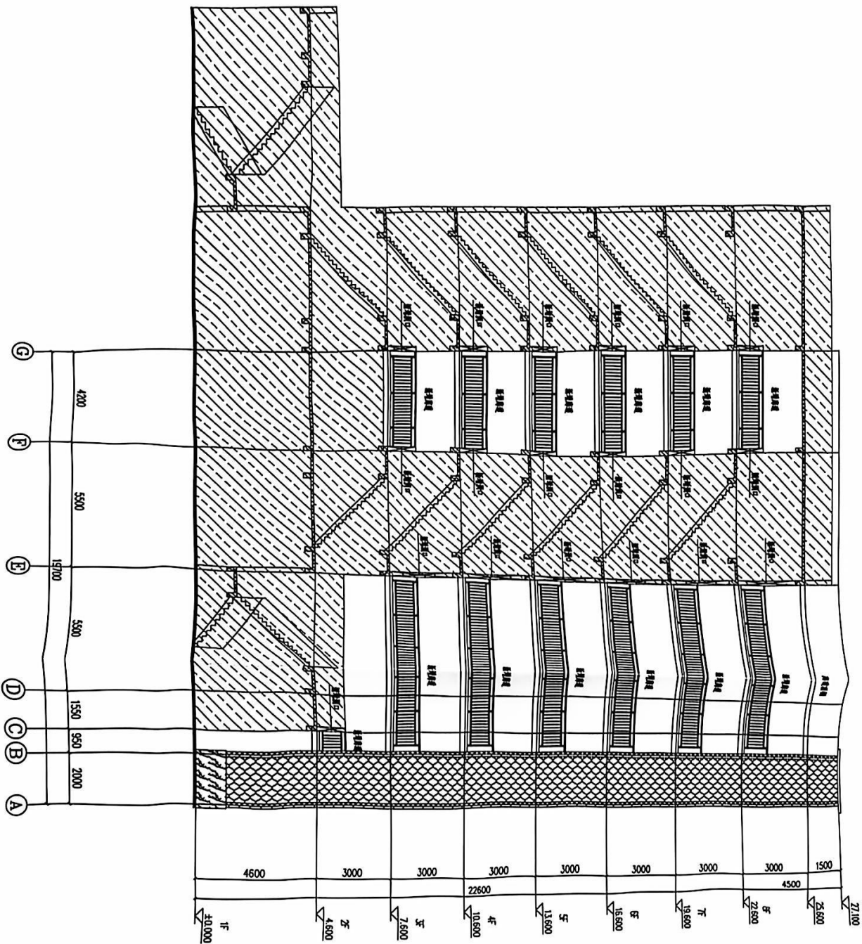
增设电梯剖面示意图
